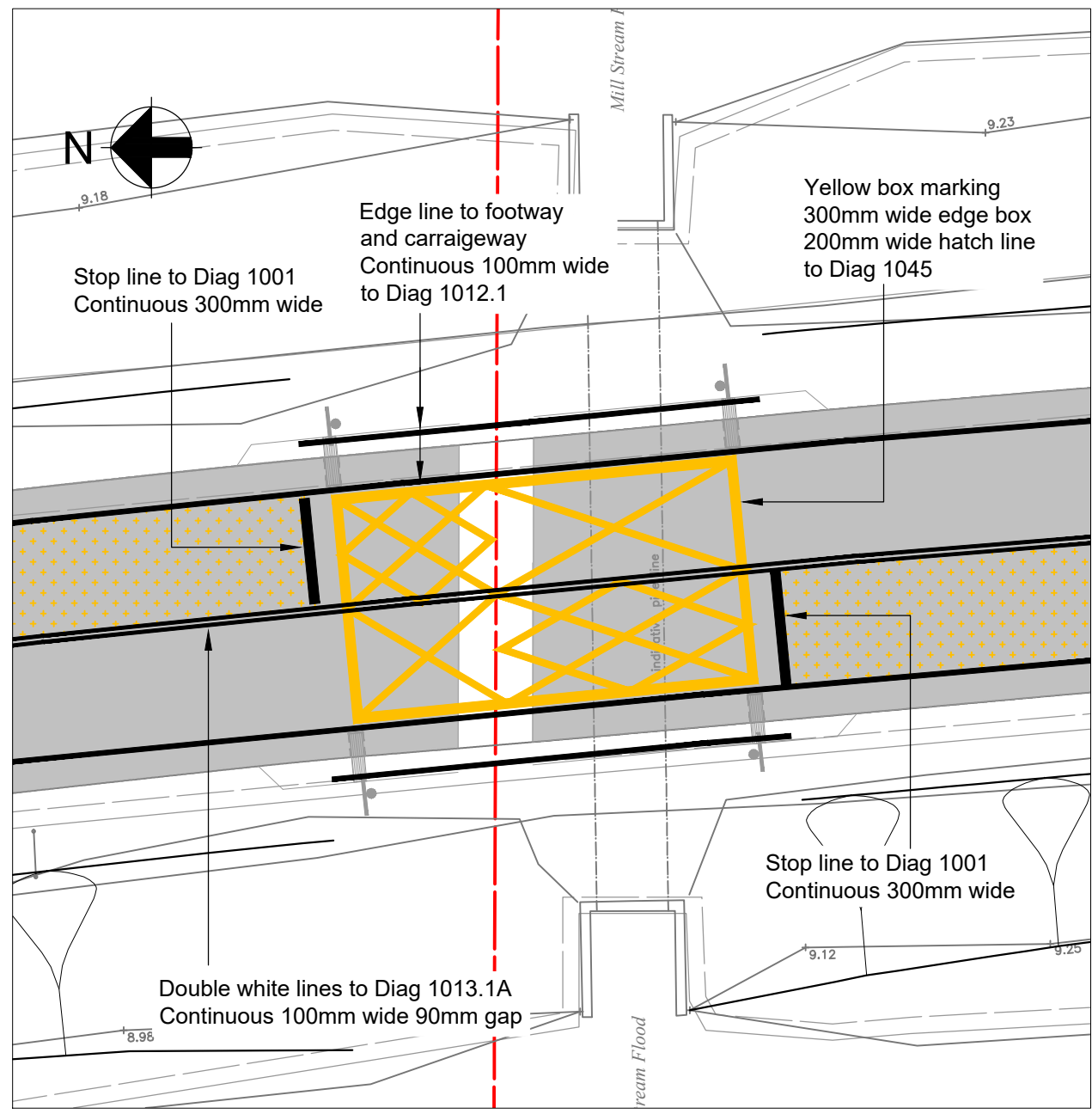
Inset A Scale: 1:250
